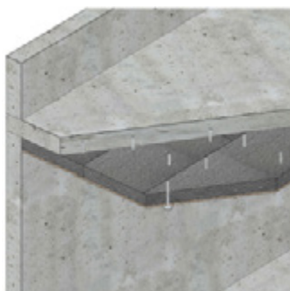
Isolation des hauts de sous-sol non chauffé avec Knauf XTherm Reno SE
