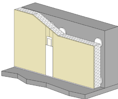
Exemple de doublage avec Polyplac (Knauf Therm Th38)
