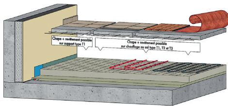
Isolation sous chape avec Knauf Thane Sol
